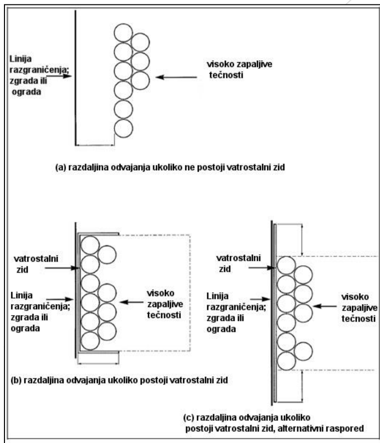
Slika 6.7.13. Pozicioniranje buradi
