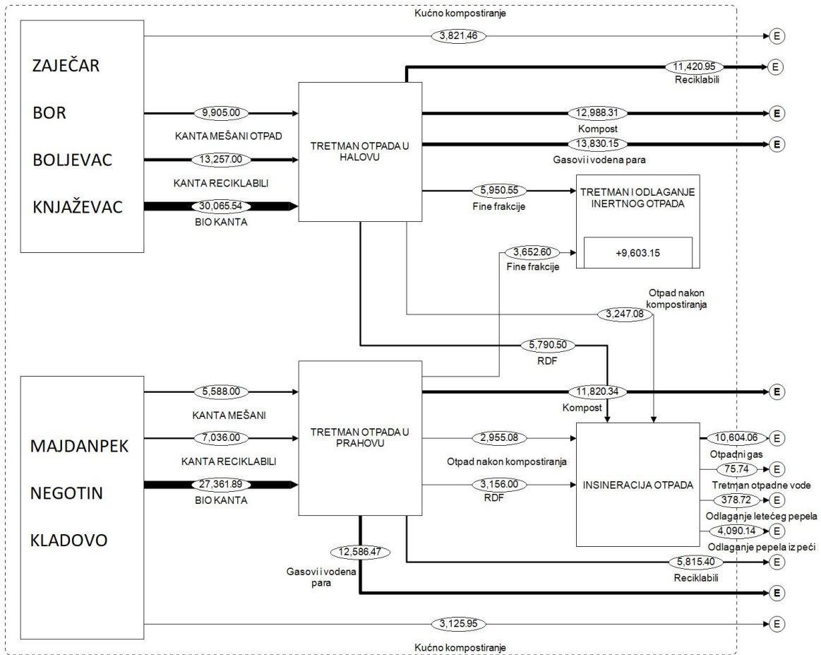
Grafik 6.4.4 Analiza tokova materijala, Model 2b – Model sakupljanja u tri kante uz povećan obuhvat sakupljanja otpada na 100% uz projekcije količina otpada do 2030. godine implementiran tretman otpada u Halovu i Prahovu, t/god
