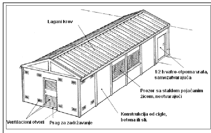
Slika 6.7.9. Vatro-otporna zgrada za skladištenje zapaljivih materijala
