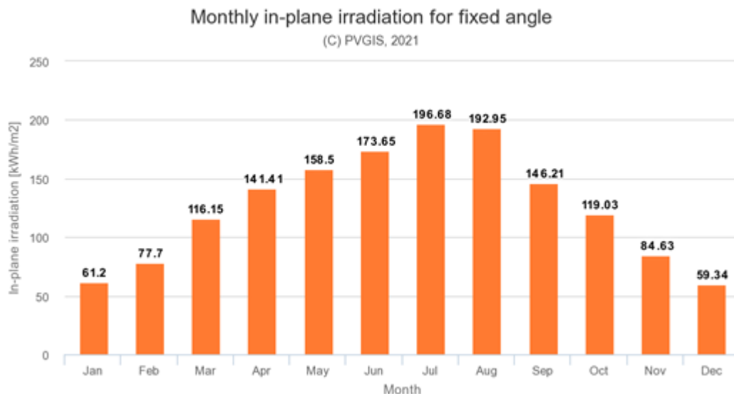
Слика број 11- Месечно зрачење сунчеве енергије са фиксним углом за село Понор
