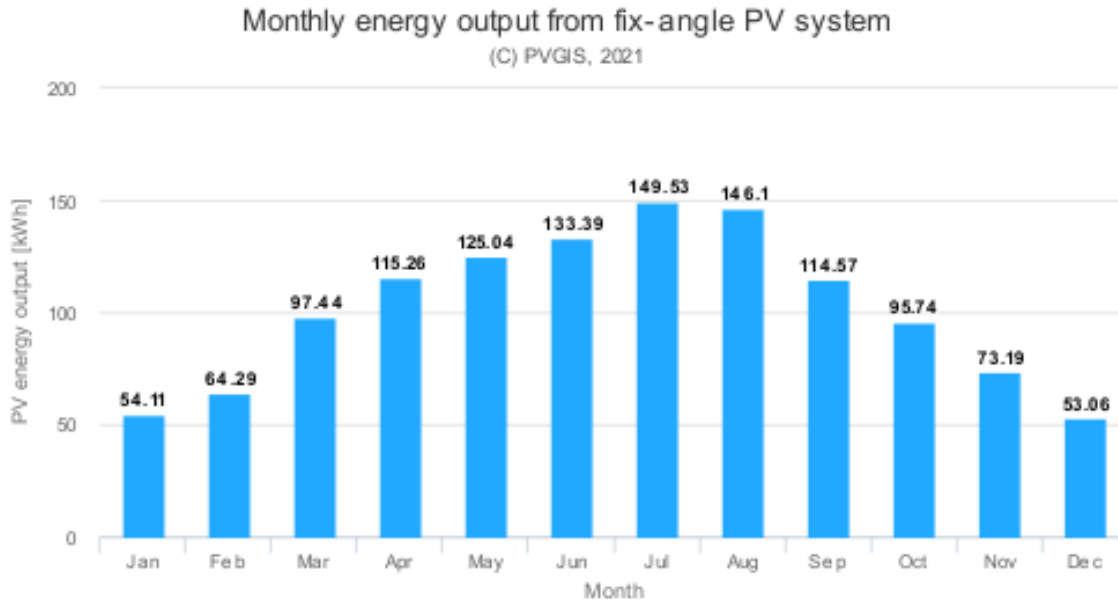
Слика број 10 - Месечни излаз енергије PV система са фиксним углом за село Понор
