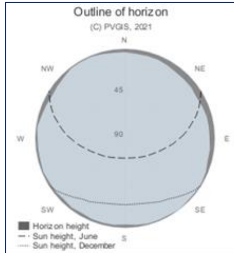
Слика број 5 - Обрис хоризонта
