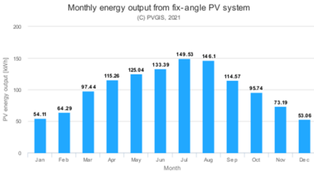
Слика број 6 - Месечни излаз енергије PV система са фиксним углом за село Понор
