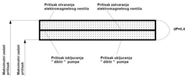
Слика 5. Шематски приказ распореда задатих притисака у микропроцесорском регулатору
