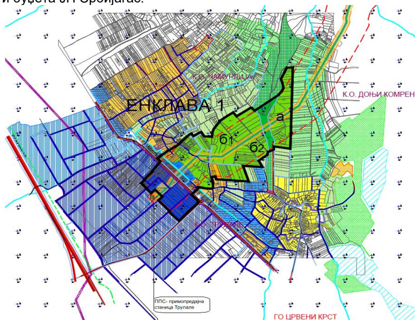
Слика 4. - План генералне регулације подручја у обухвату заштитног појаса инфраструктурног коридора магистралног гасовода Ниш-Димитровград (Приказ: ППС- примопредајна станица Трупале)
