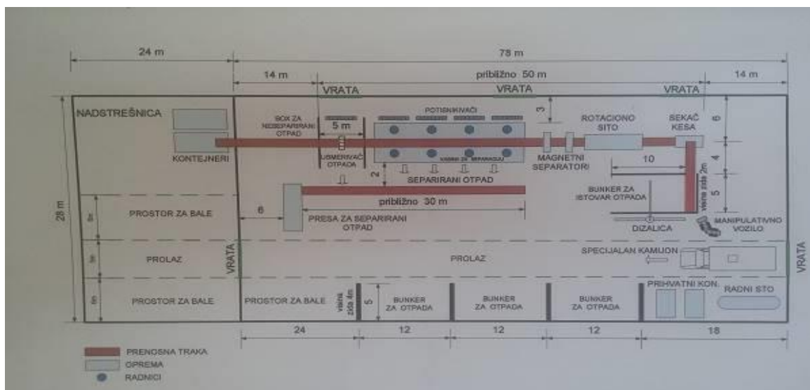
Слика 5.14 Шема постројења за сепарацију и балирање отпада
